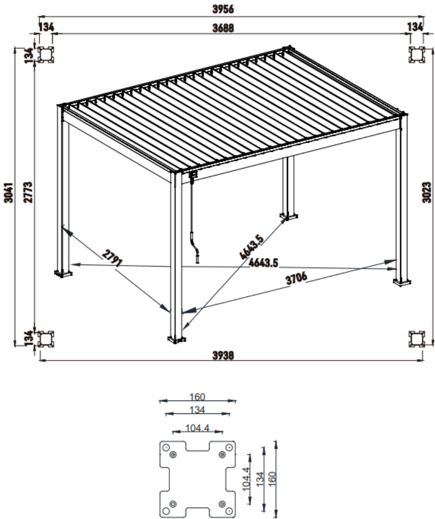
Plan de montage (dimensions en mm)
